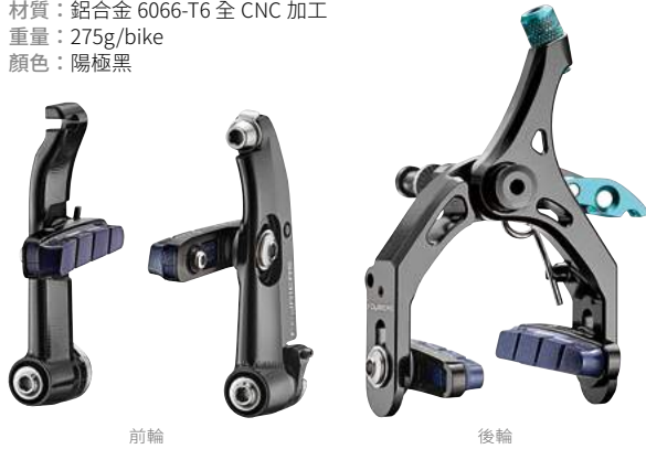
前輪
