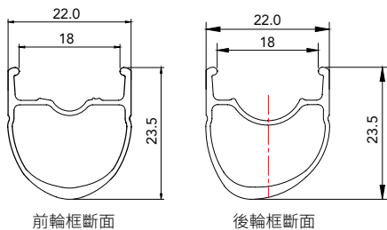
前輪框斷面
